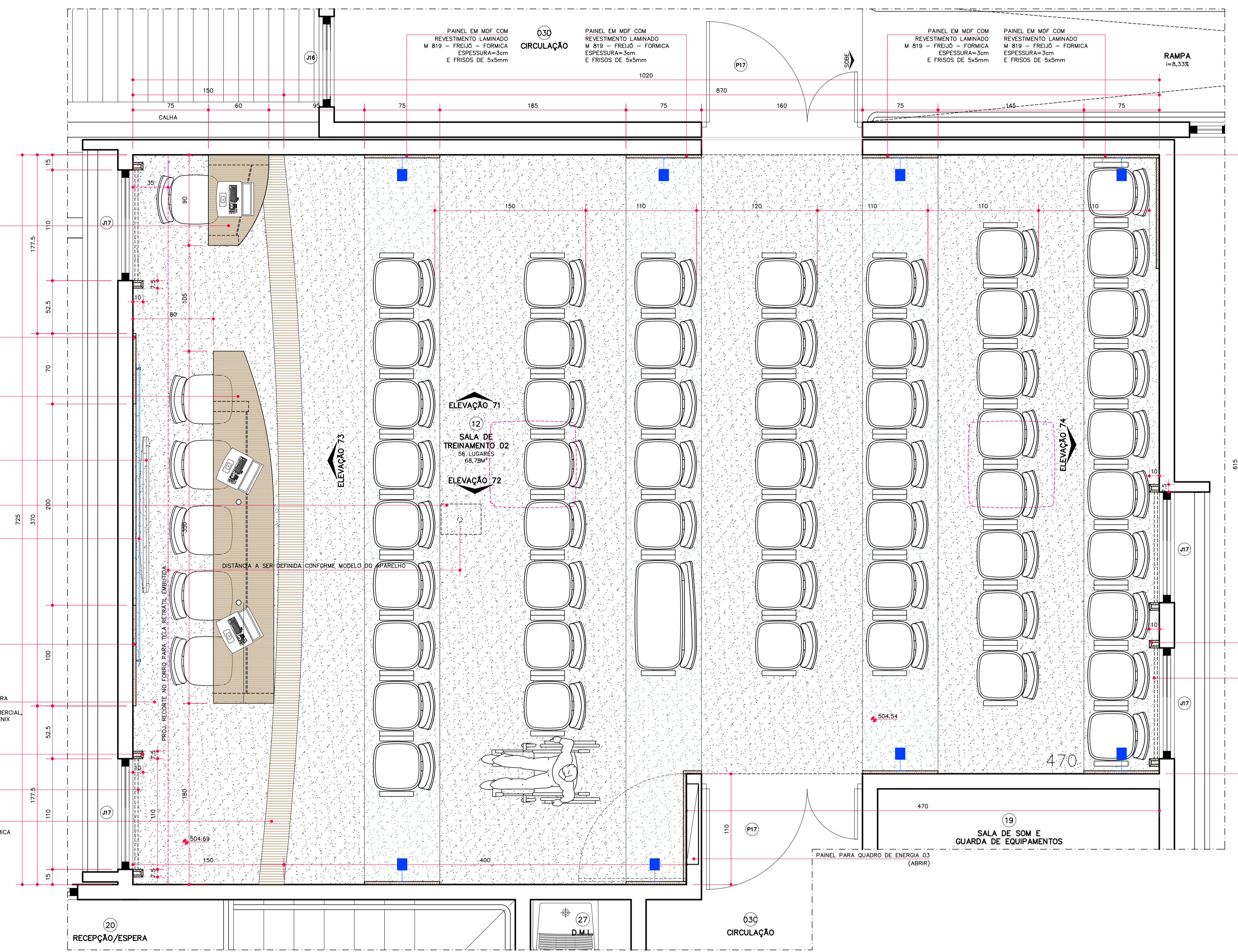
PLANTA SALA DE TREINAMENTO 02 (12) 1:25
