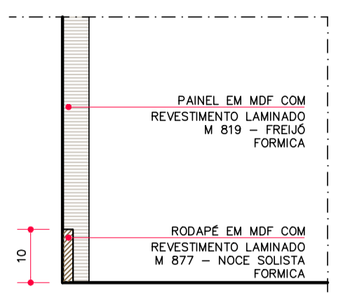
DET. 21 - RODAPÉ EM MDF 1:10
